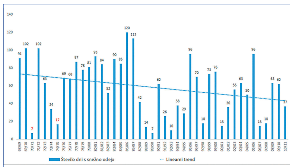
Slika 63: Število dni s snežno odejo v snežnih sezonah v Livku v obdobju 1968–2011. Za snežni sezoni 70/71 in 74/75 (rdeči številki) vsi podatki niso na voljo. Razvidno je upadanje števila dni s snežno odejo. (Vir podatkov: Arhiv meteoroloških podatkov, 2020)
